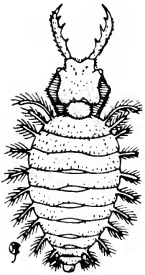
Fig. 397. Ulu-lodes hyalina Latr.
